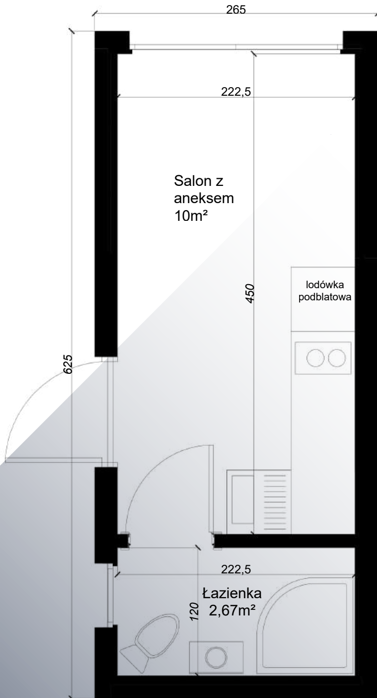
RZUT PRZYZIEMIA
