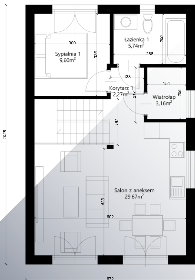
RZUT PARTERU
