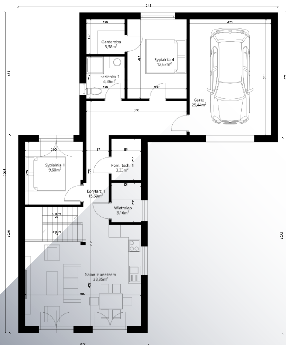
RZUT PARTERU
