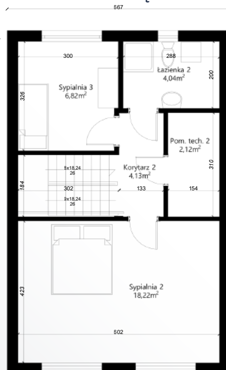
RZUT PIĘTRA
