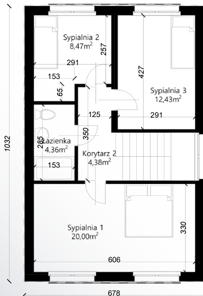
RZUT PIĘTRA
